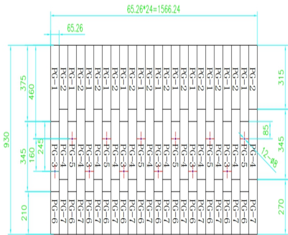
上升浸渍管展开图
